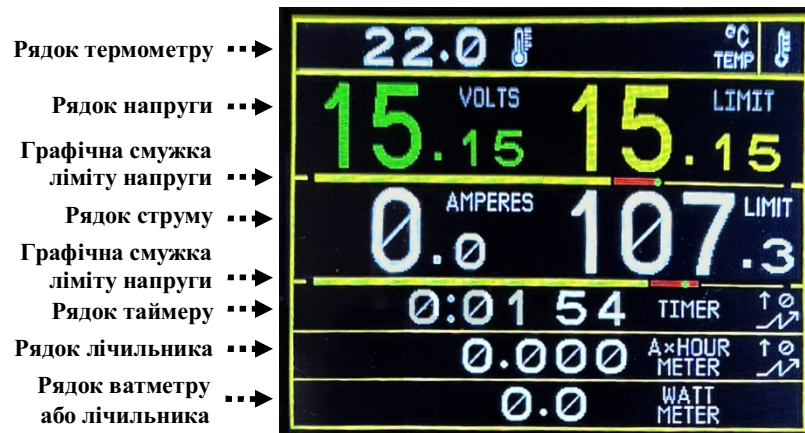
Мал. 3. Відображення інформації на дисплеї джерела живлення
