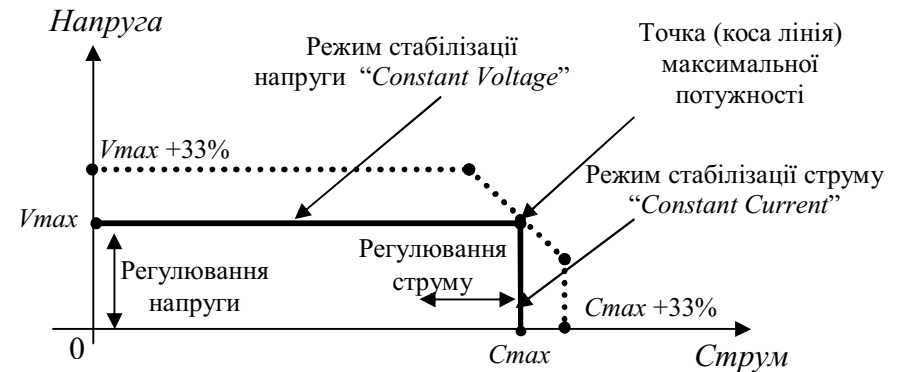
Мал. 17. Вольт-амперна характеристика джерела живлення
