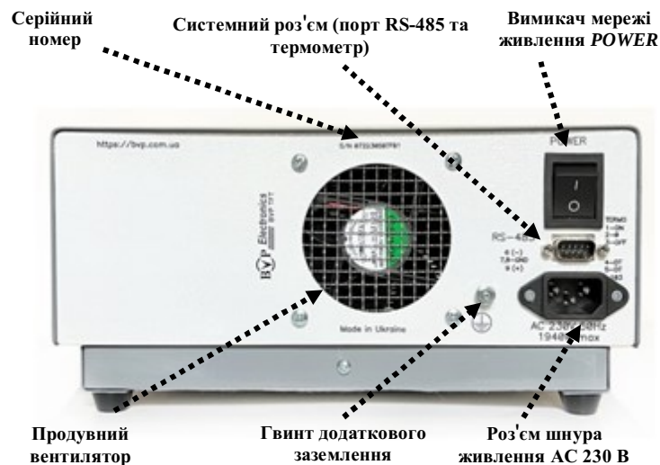
Мал. 4. Задня панель джерела живлення
