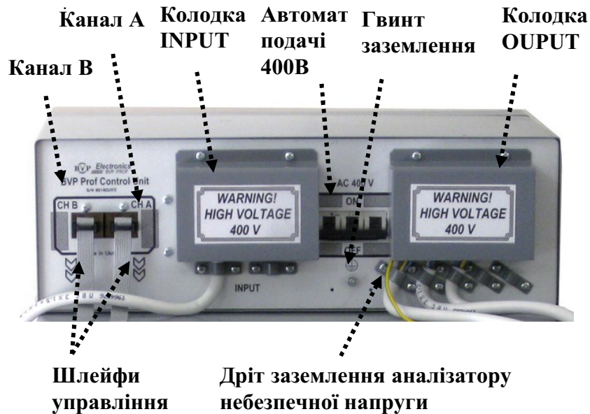
Мал. 4. Зовнішній вигляд задньої частини блоку управління
