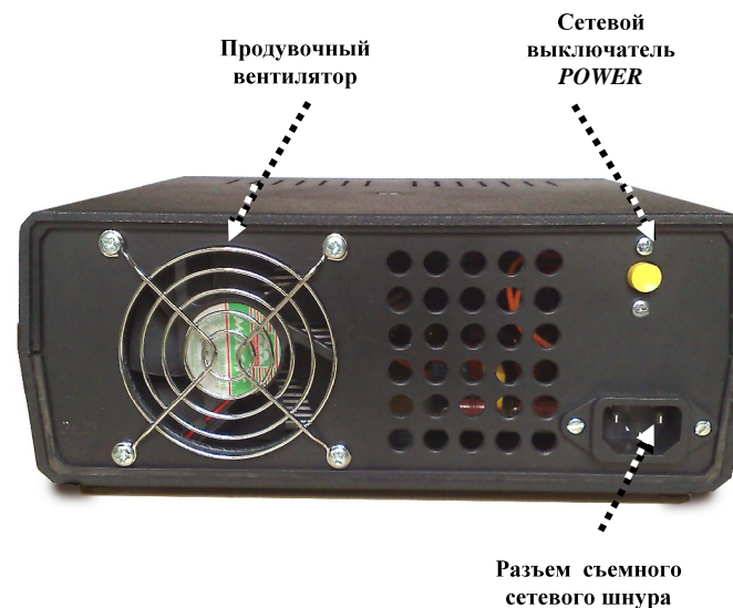
Рис. 3. Расположение органов управления на задней панели источника питания
