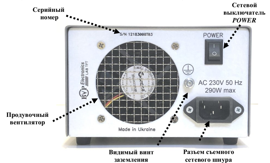
Рис. 3. Расположение органов управления на задней панели источника питания
