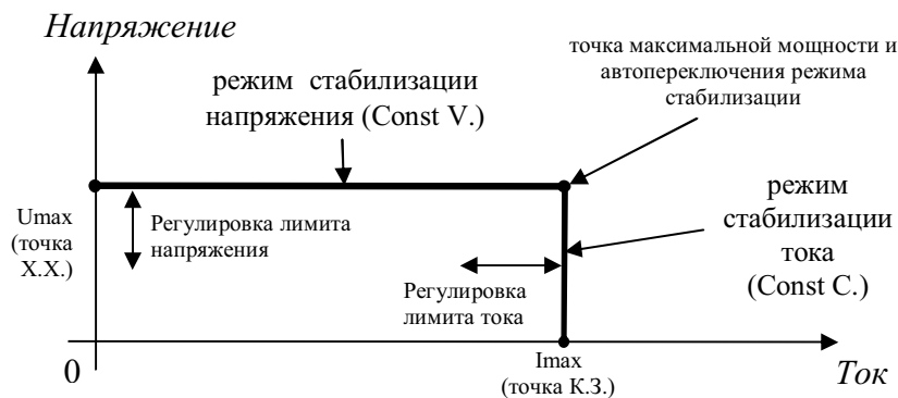
Рис. 2. Вольт-амперная характеристика источника питания
