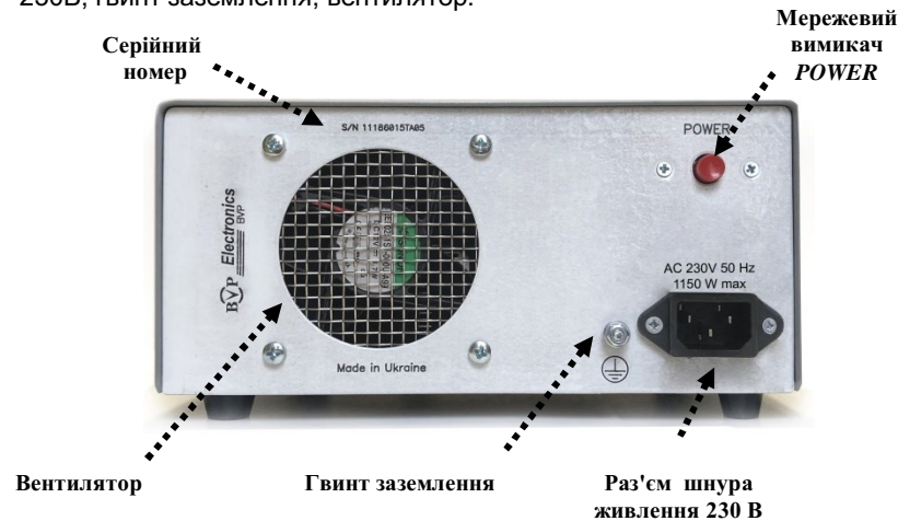
Мал. 3. Розташування органів управління на задній панелі джерела живлення
