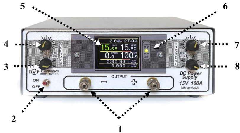
Мал. 2. Розташування органів управління на передній панелі джерела живлення
