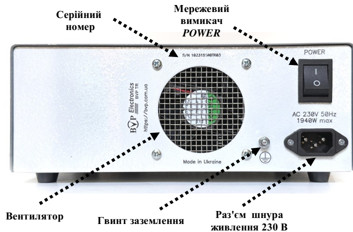
Мал. 3. Розташування органів управління на задній панелі джерела живлення
