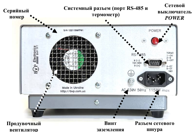
Рис. 4. Задняя панель источника питания
