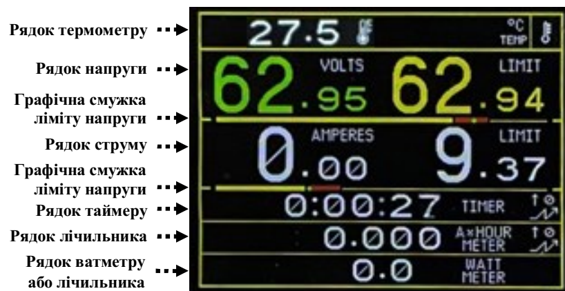
Мал. 3. Відображення інформації на дисплеї джерела живлення
