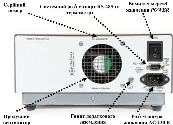
Мал. 4. Задня панель джерела живлення
