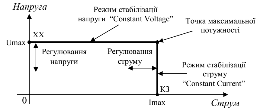
Мал. 17. Вольт-амперна характеристика джерела живлення
