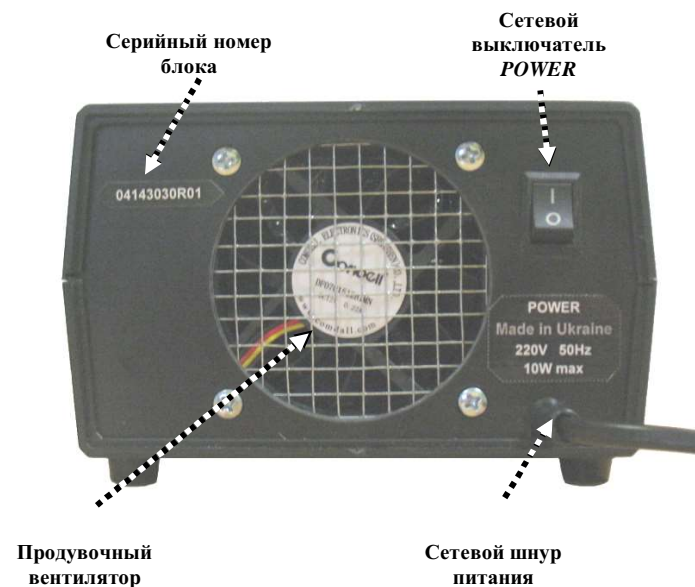
Рис. 3. Расположение органов управления на задней панели блока
