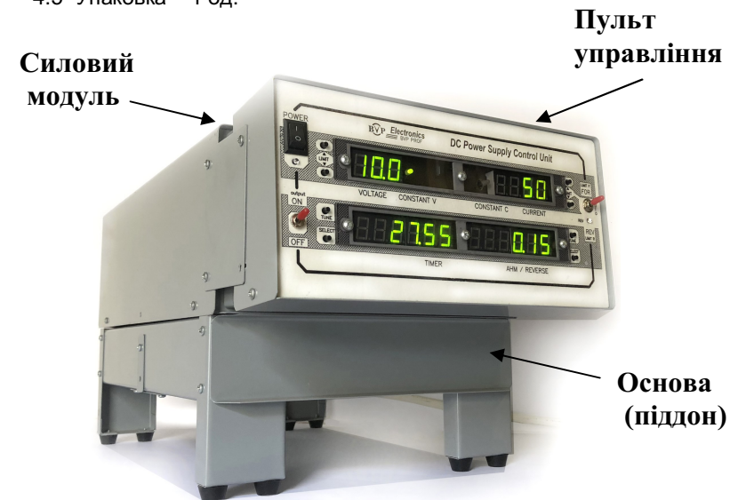
Мал. 2. Складові частини випрямляча
