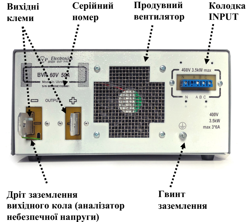
Мал. 6. Зовнішній вигляд задньої панелі силового модуля
