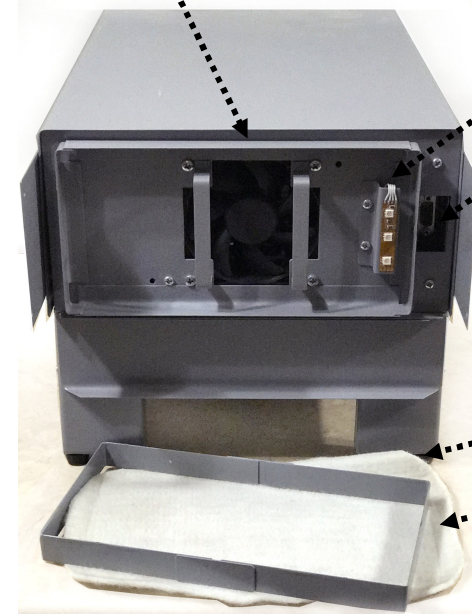
Мал. 5. Передня панель силового модуля без фільтру
