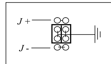
Рис. 7 Снятие заземления с выходных клемм источника
