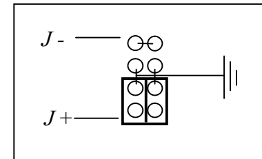
Рис. 6 Заземление плюсовой клеммы
