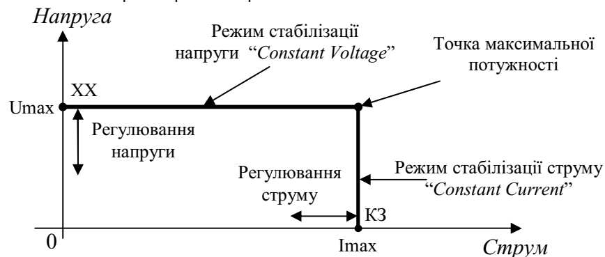
Мал. 5. Вольт-амперна характеристика джерела живлення
