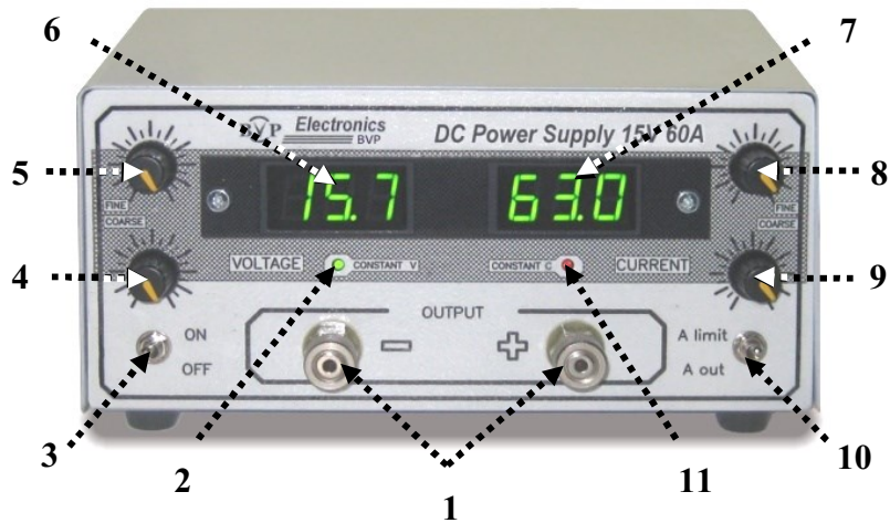
Мал. 2. Розташування органів управління на передній панелі джерела живлення
