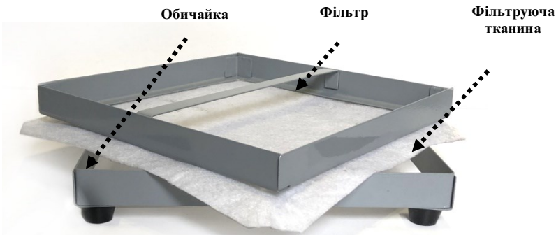
Мал. 4. Повітряний фільтр
