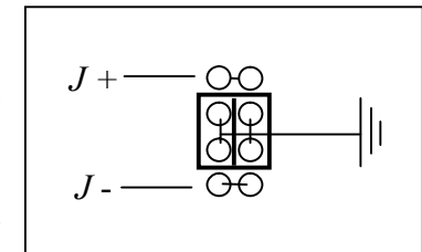
Рис. 14 Снятие заземления с выходных клемм источника
