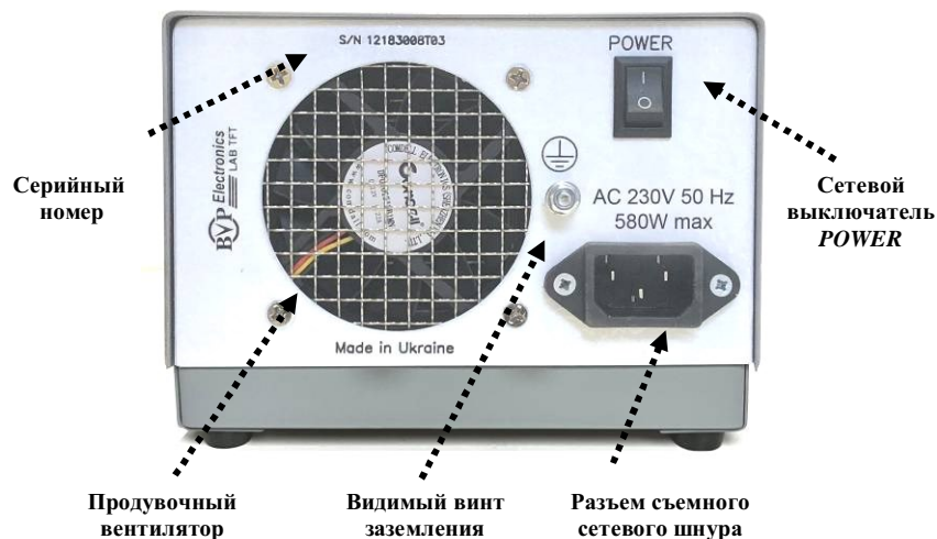
Рис. 4. Расположение органов управления на задней панели источника питания
