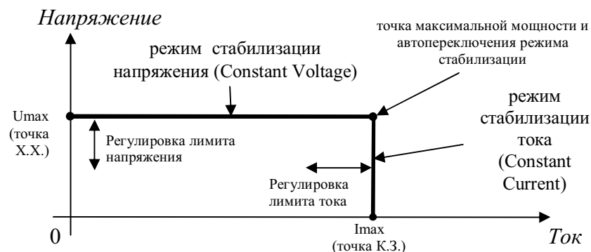
Рис. 16. Вольт-амперная характеристика источника питания
