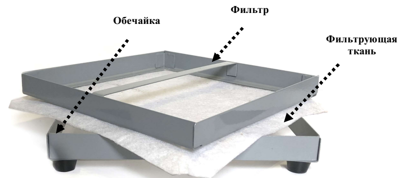
Рис. 5. Съемный воздушный фильтр
