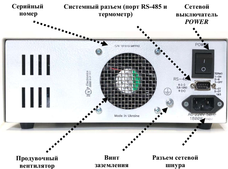
Рис. 4. Задняя панель источника питания
