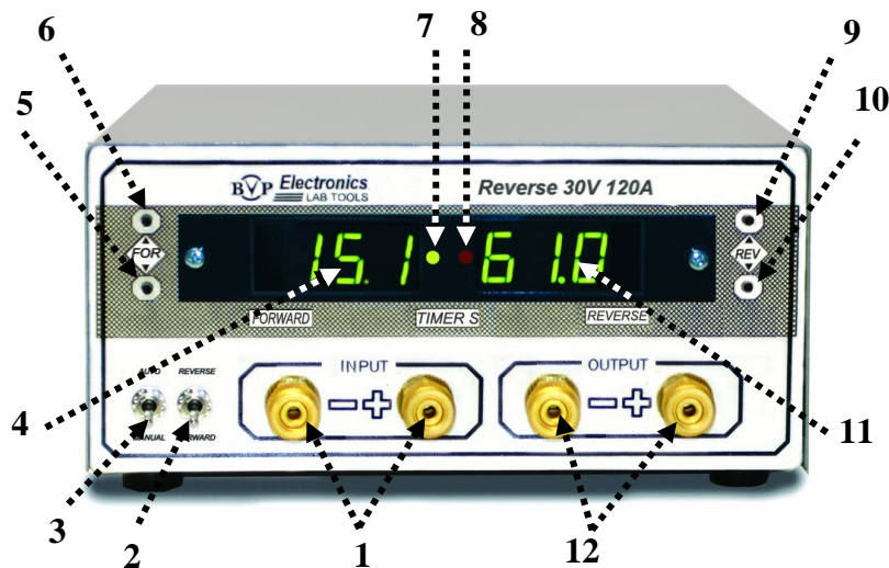
Рис. 2. Расположение органов управления на передней панели блока реверсного переключения тока
