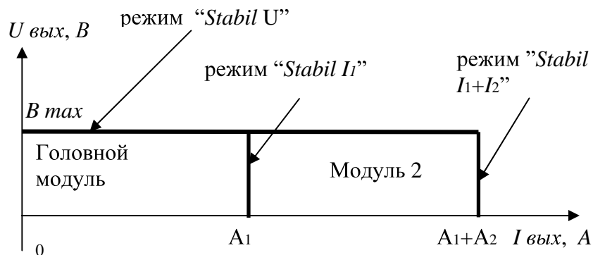
Рис. 6 Вольт-амперная характеристики при параллельном подключении модулей
