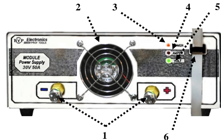
Рис. 3. Расположение органов управления на передней панели управляемого модуля источника питания
