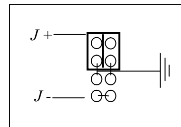
Рис. 13 Заземление плюсовой клеммы
