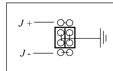
Рис. 14 Снятие заземления с выходных клемм источника
