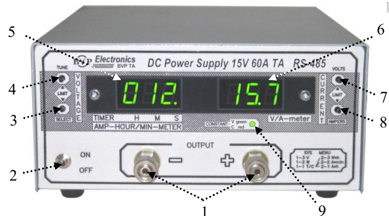
Рис. 2. Расположение органов управления на передней панели источника питания
