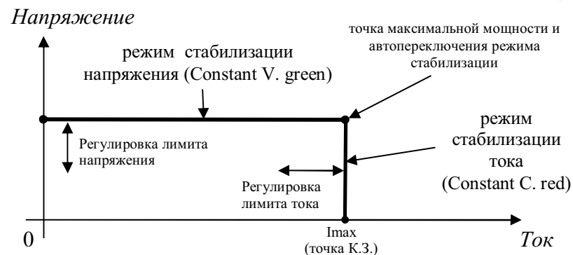
Рис. 11. Вольт-амперная характеристика источника питания
